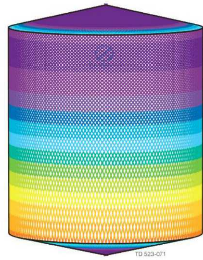
D4,6m H5,5m, Toftejorg TJ 20G, 4 x ø5.5 mm, Tempo = 8.3 min., consumo acqua = 1612 l
