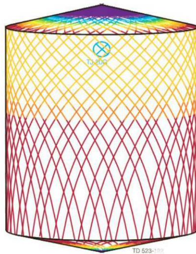
D4,6m H5,5m, Toftejorg TJ 20G, 4 x ø5.5 mm, Tempo = 2.08 min., consumo acqua = 403 l
