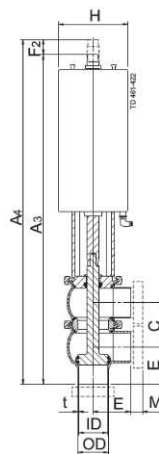
Valvola deviatrice
